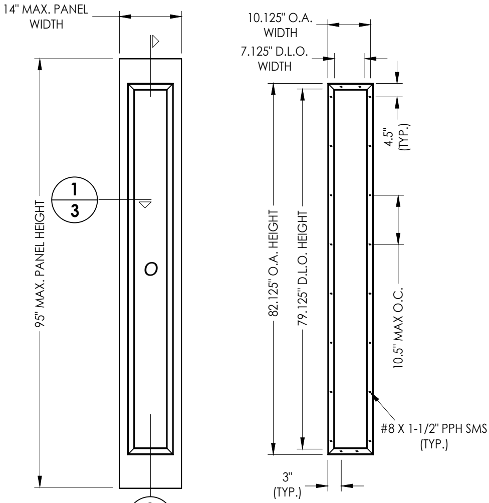
ODL LITE FRAME
